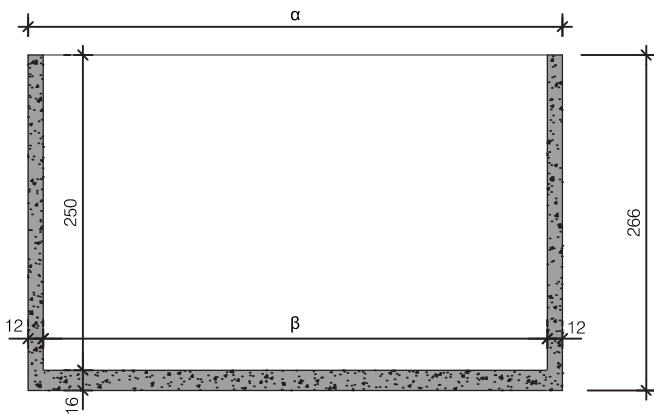
Langdoorsnede
