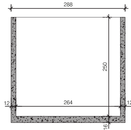
Dwarsdoorsnede
